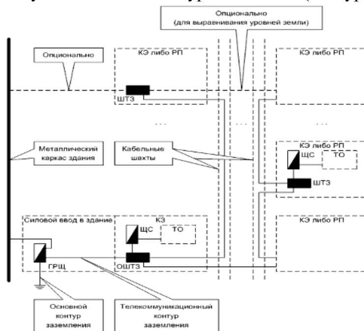
Модель заземления
